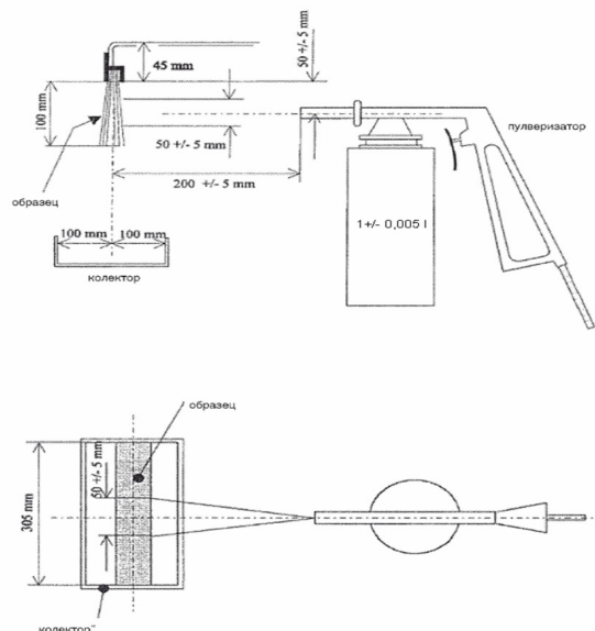
Фиг. 2. Изпитвателен стенд за устройства против изпръскване от типа сепаратор въздух/вода.
