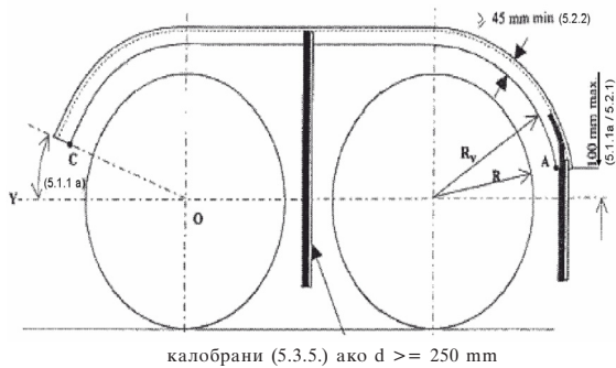
Фиг. 4. Диаграма, показваща комплект система против изпръскване (калник, калобран, външна престилка), включваща устройства против изпръскване (енергийно-абсорбиционен тип) при многоосие.
