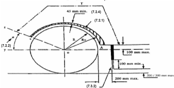
Фиг. 5. Диаграма, показваща комплект система против изпръскване, включваща устройства против изпръскване (енергийно-абсорбиционен тип) за оси, оборудвани с неуправляеми или самоуправляеми колела (т. 4.2 и 6 на част I и II).
