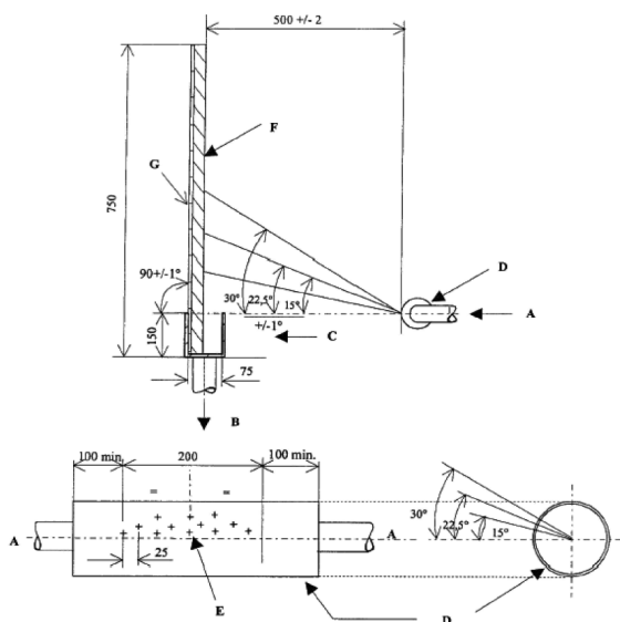
Фиг. 1. Изпитвателен стенд за устройство против изпръскване от енергийно-абсорбционен тип.
