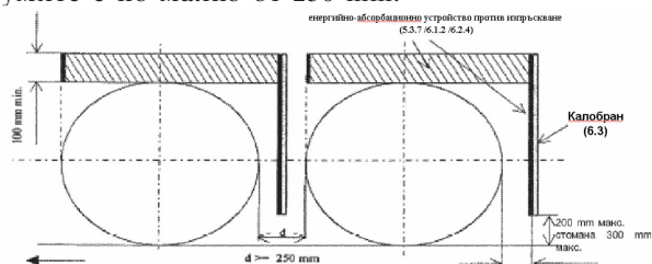
б) Единични оси или многоосие, където разстоянието между гумите е не по-малко от 250 mm.
