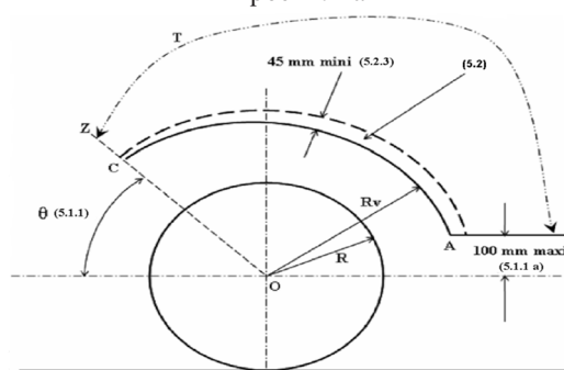
Фиг. 1б. Пример за измерване на външната престилка
