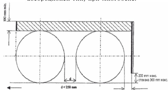
а) Многоосие, където разстоянието между гумите е по-малко от 250 mm.
